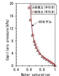
図2 水分特性曲線
