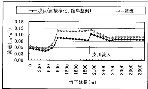
図-4 事業実施後の流速
