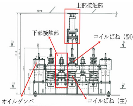
図-4 IMD構造図
