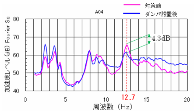
図-11 床版振動周波数分析図
