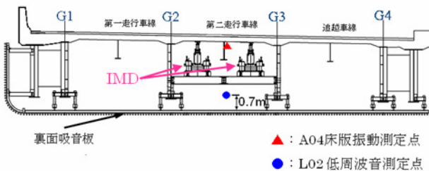
図-9 IMD配置図(横断図)
