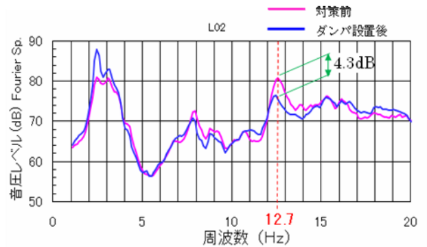
図-12 低周波音周波数分析図
