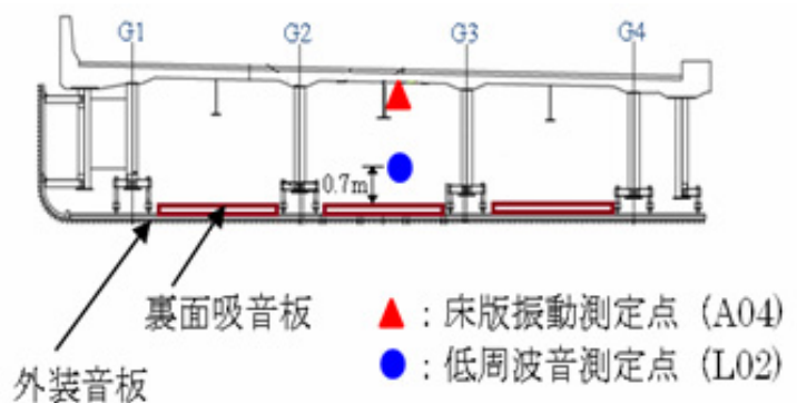
図-6 横断面図
