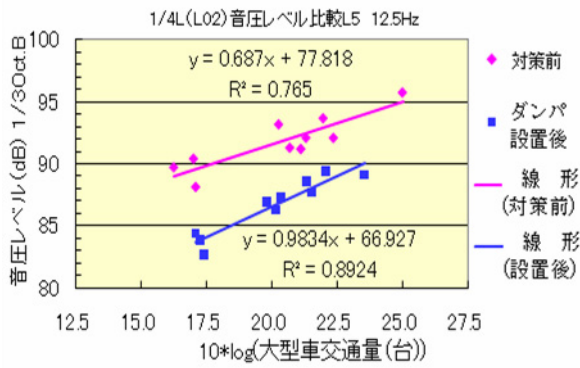
図-13 大型車交通量別の効果 (低周波音)
