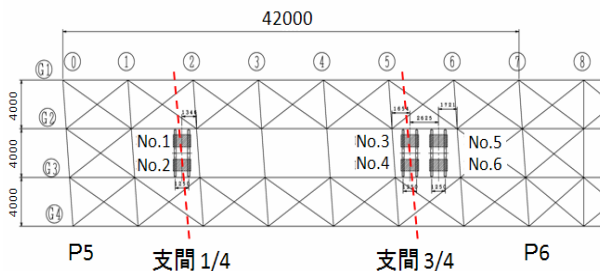
図-10 IMD配置図(平面図)
