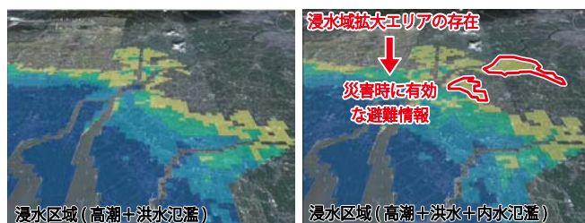
図3 氾濫解析結果例(内水氾濫考慮有無による比較)
