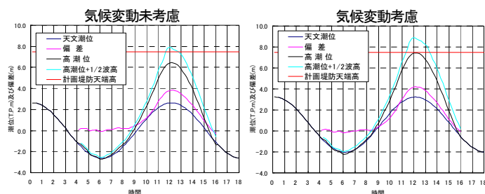
図2 高潮予測結果(潮位および偏差・波高の時系列変化)
