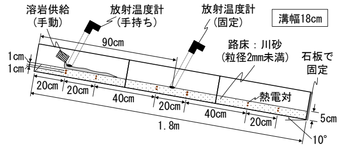
図-1 小型流路の模式図
