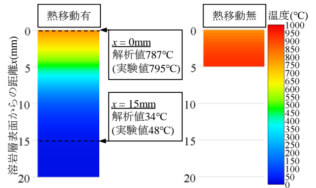
図-5 温度分布の解析結果(経過時間 30 秒)
