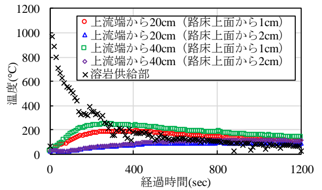
図-3 路床温度と溶岩供給部温度の時系列変化(10 秒間隔)
