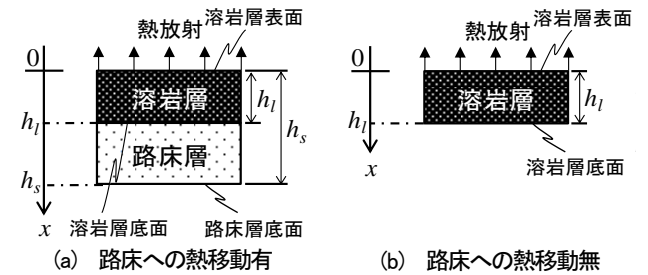
図-4 解析モデル 4)
