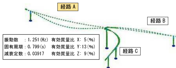
図7 鉛直方向卓越モード図（1次モード）
