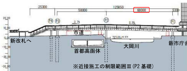
図4 主橋梁部(渡河部)の支間割
