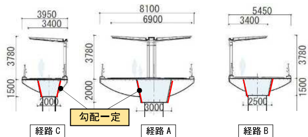
図6 各径路の桁断面と桁高変化
