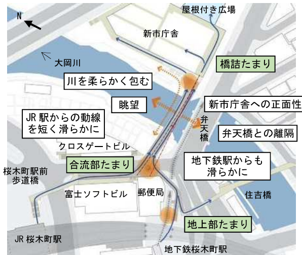
図2 平面線形の考え方
