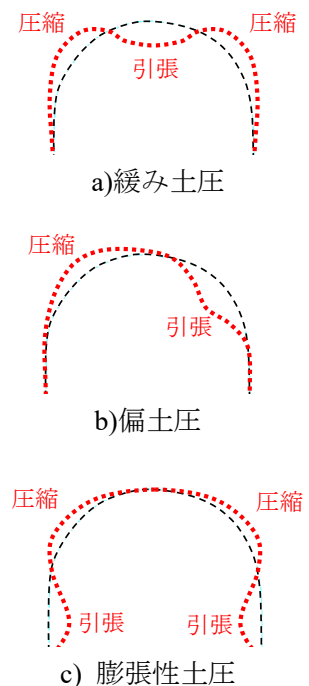
図-2 変形モードによる土圧の推定 1)
