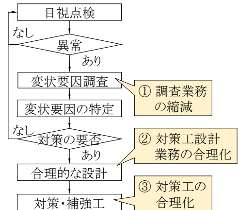
図-1 光ファイバ計測技術によるトンネル維持管理の生産性向上の効果
