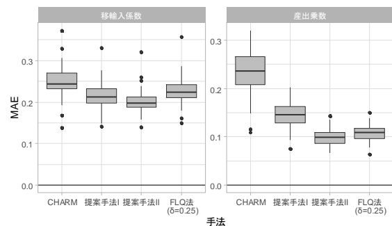
図-6 従来手法と提案手法の精度比較
