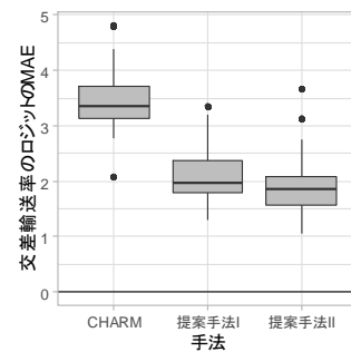
図-5 交差輸送率の精度比較（都道府県表）
