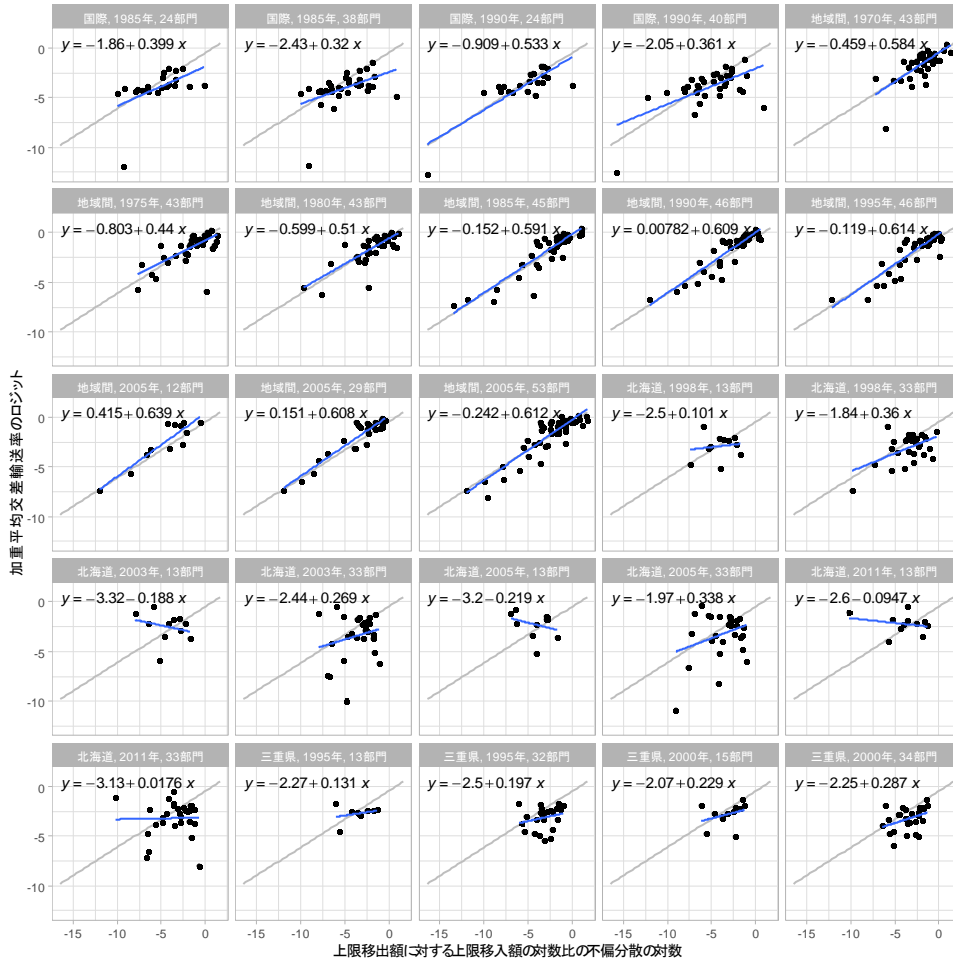
図-2 地域間産業連関表別の上限移出入額分散と交差輸送率の関係 (青線：表別の回帰直線，灰色線：提案手法Iの回帰直線)
