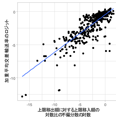
図-1 上限移出入額分散と交差輸送率の関係
