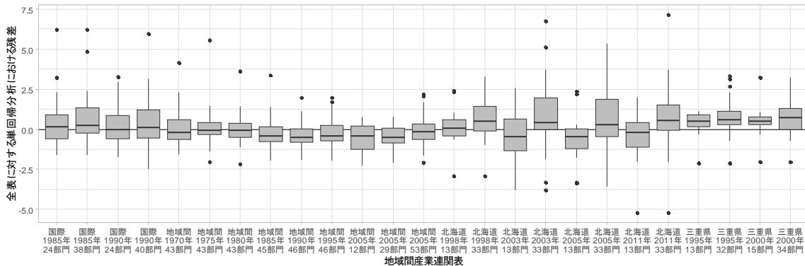
図-3 地域間産業連関表別の全表に対する単回帰分析における残差
